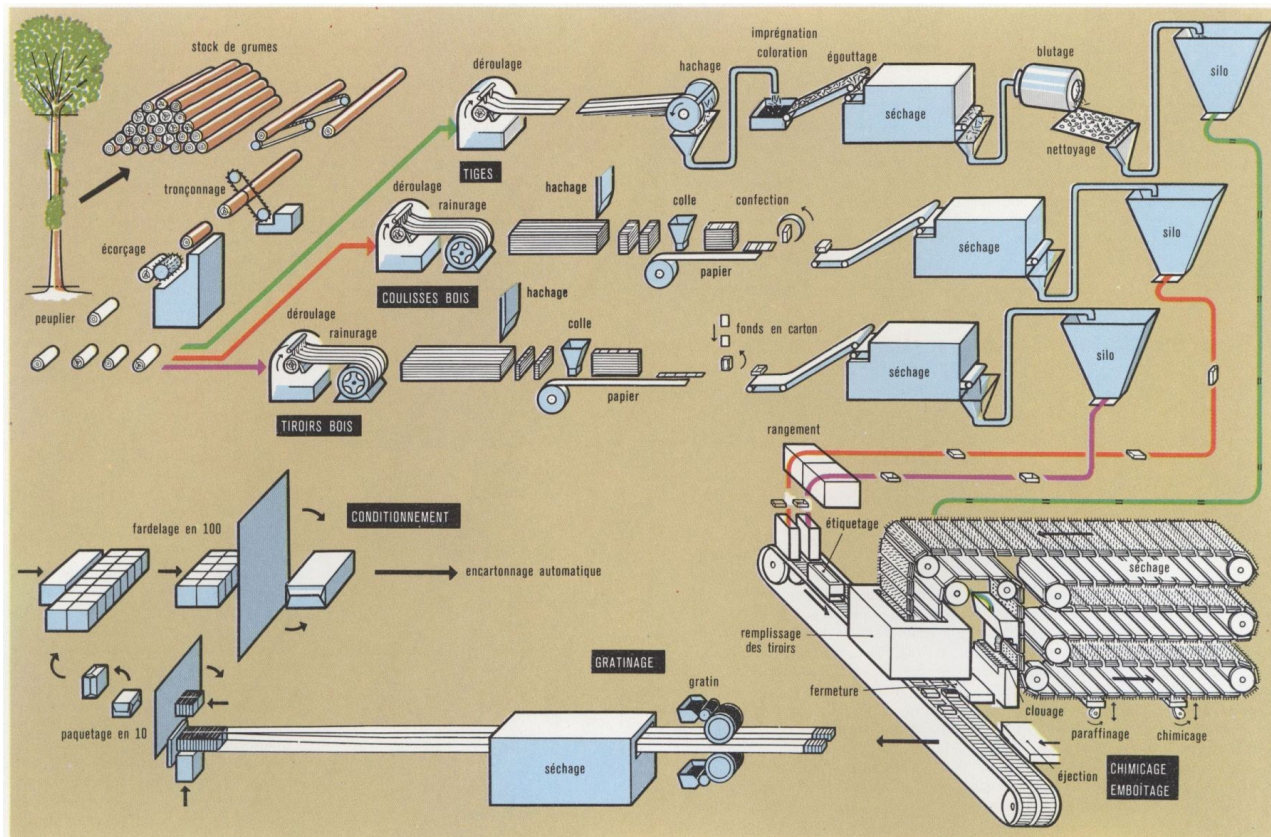
Fabrication de boîtes d'allumettes en bois.
